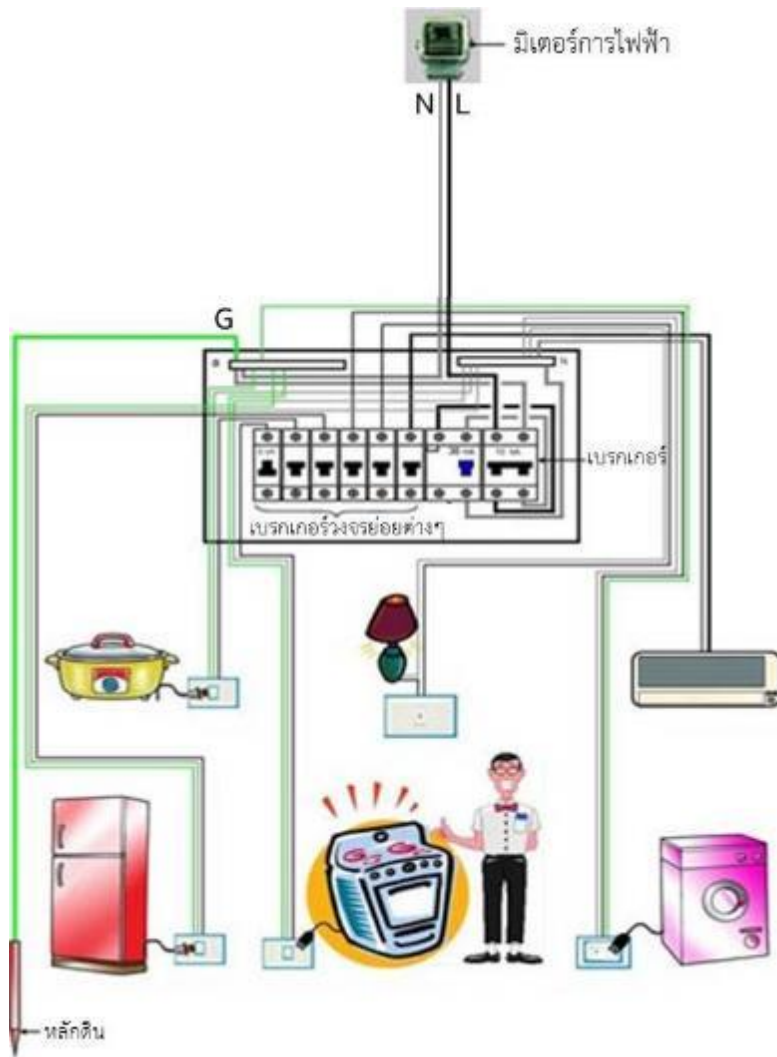
ภาพตัวอย่างแผนวงจรไฟฟ้าในครัวเรือน
