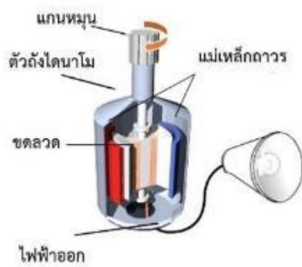
ภาพอุปกรณ์ที่มีการใช้ไฟฟ้าที่เกิดจากพลังงานแม่เหล็กไฟฟ้า
